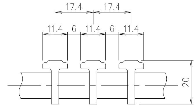
メンバー詳細図 S=1/1
