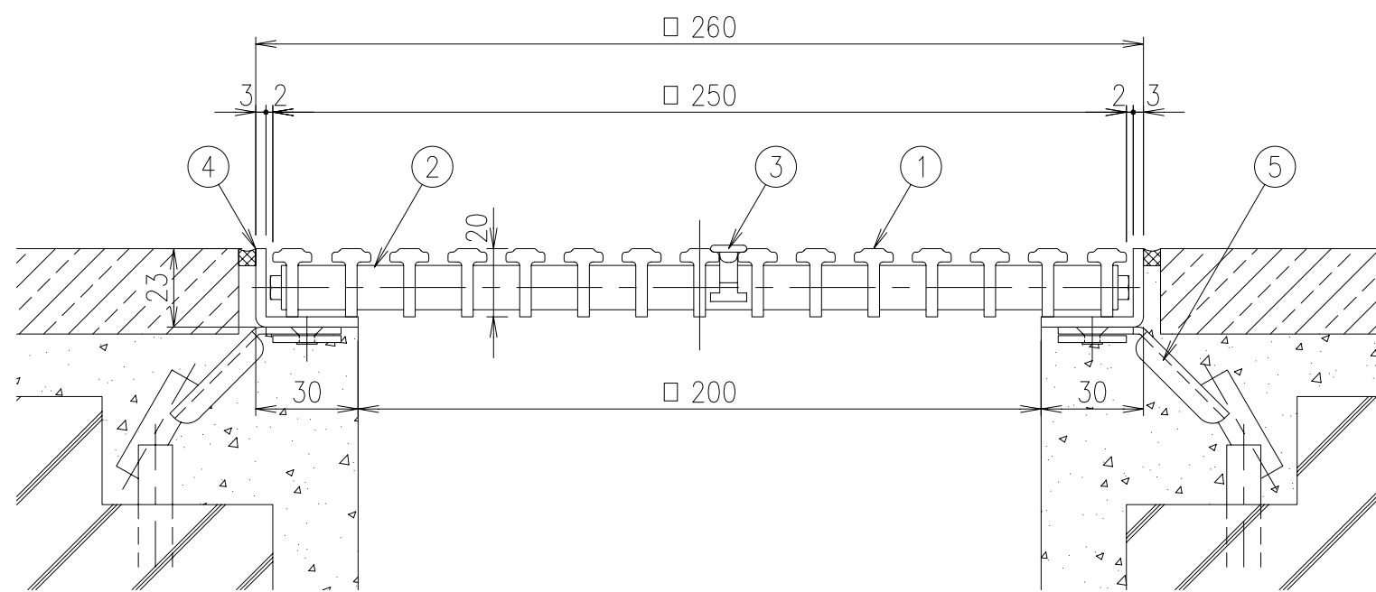
SFG-M-2025 (B・G・P・A・S・M・D・K) 断面詳細図 S=1/2
