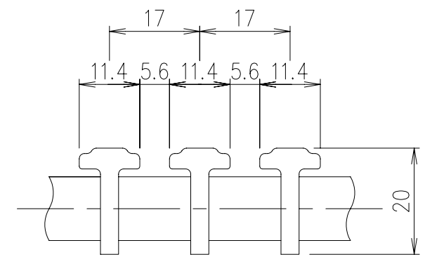
メインバー詳細図 S=1/1
