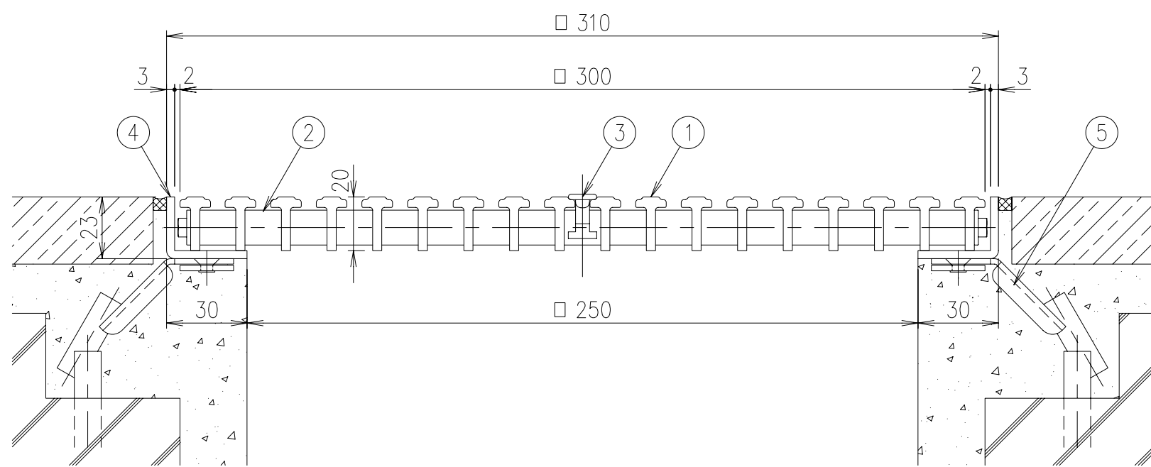
SFG-M-2030 (B・G・P・A・S・M・D・K) 断面詳細図 S=1/2
