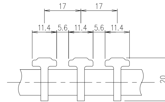
メンバー詳細図 S=1/1
