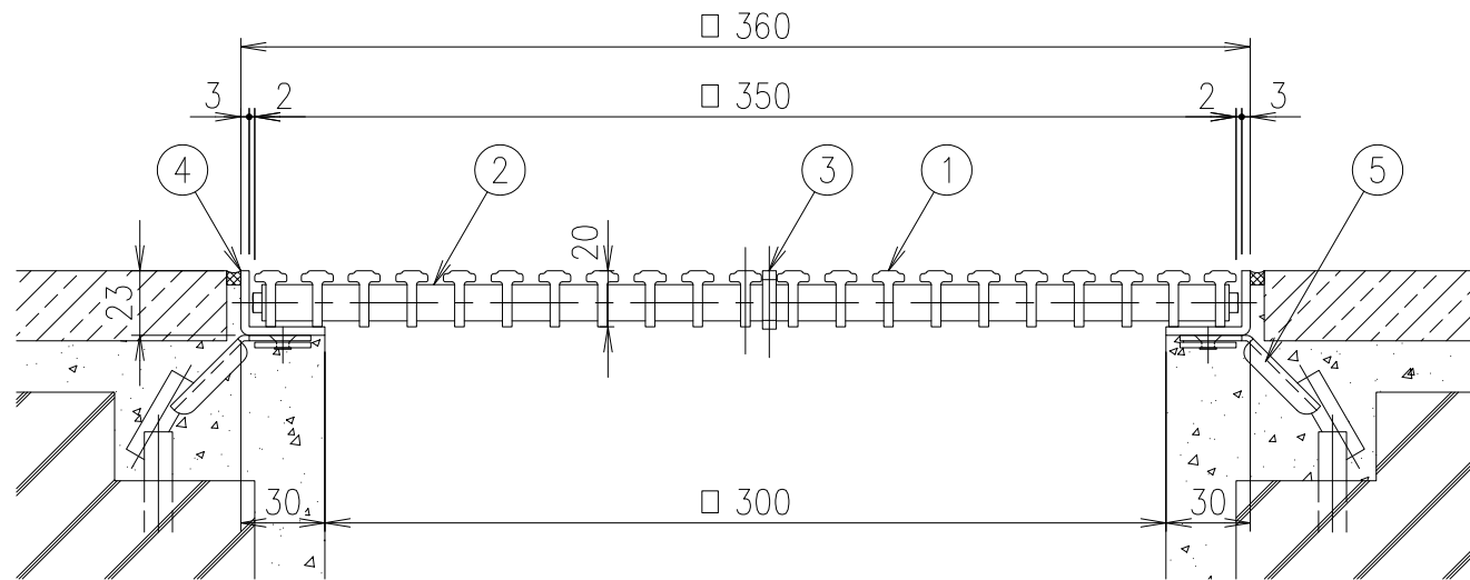
SFG-M-2035 (B・G・P・A・S・M・D・K・C) 断面詳細図 S=1/3
