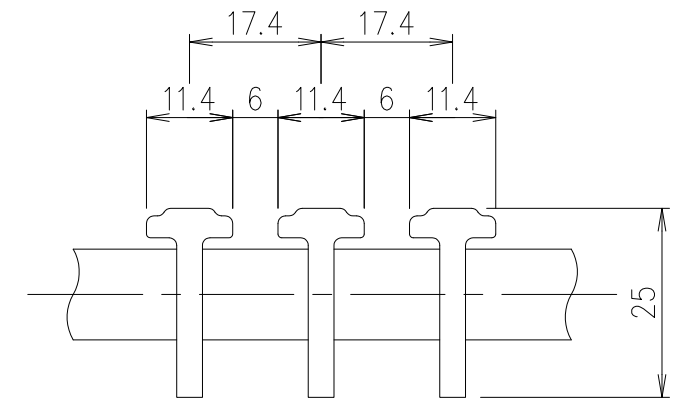
メンバー詳細図 S=1/1
