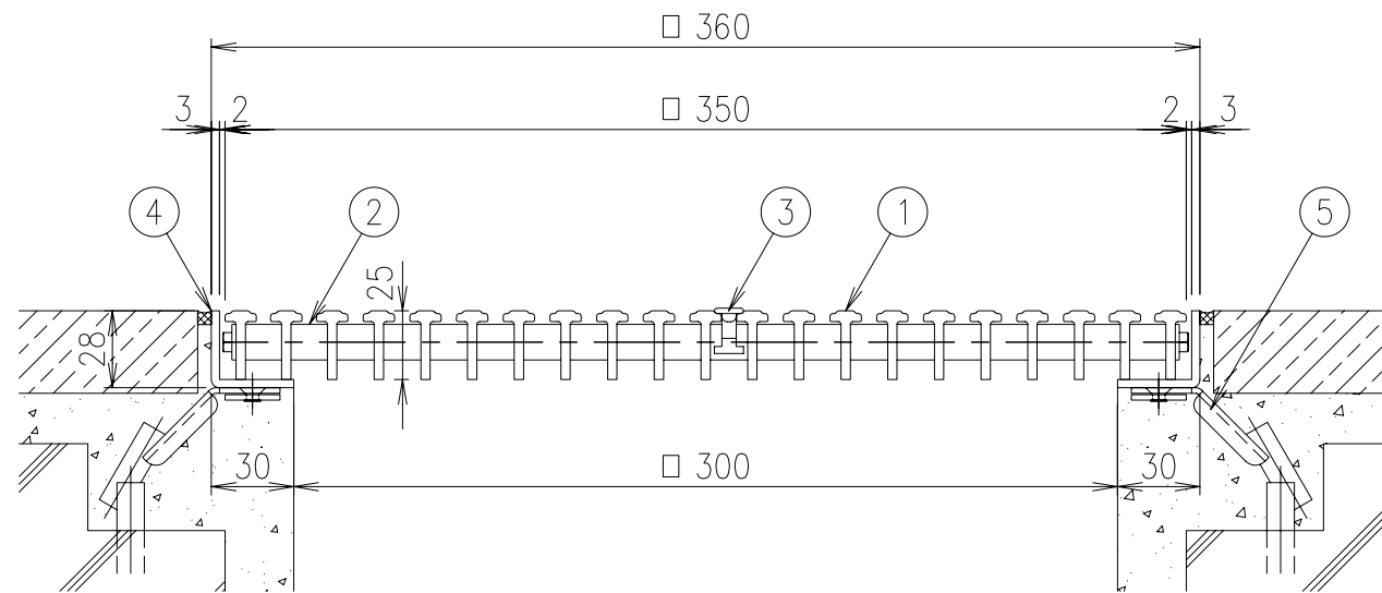
SFG-M-2535 (B・G・P・A・S・M・D・K) 断面詳細図 S=1/3
