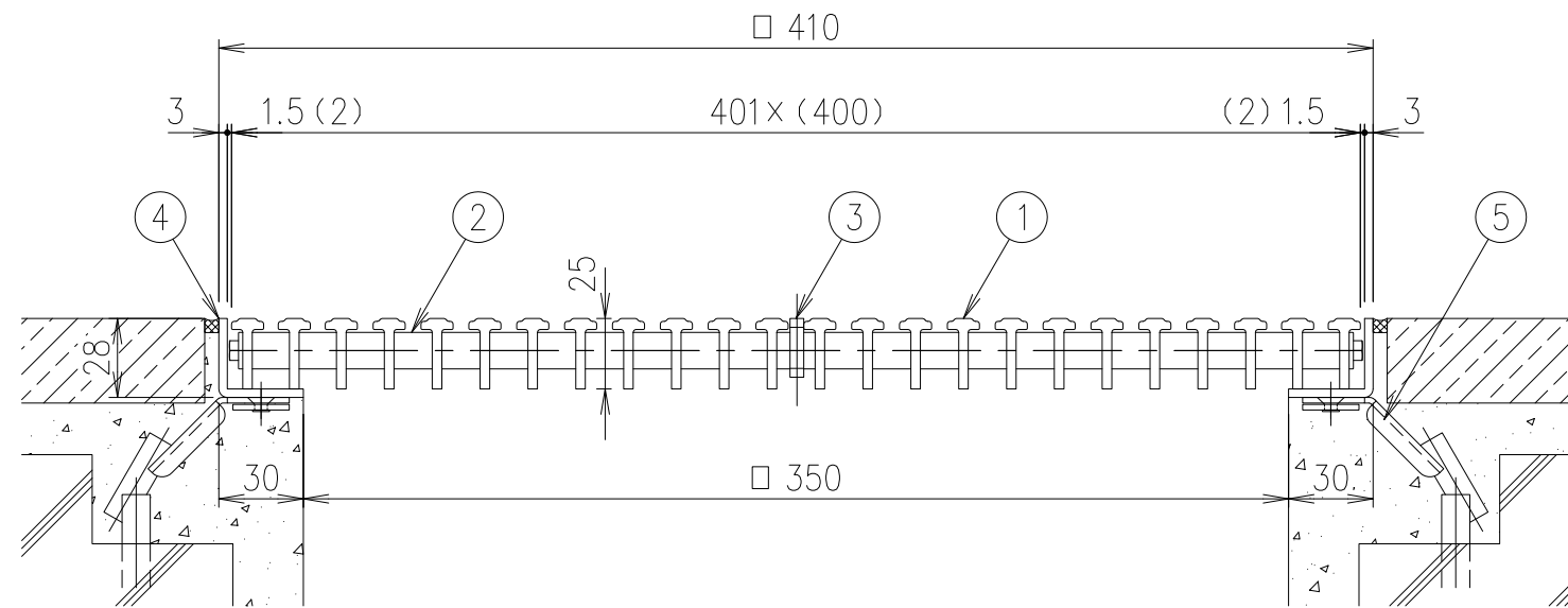
SFG-M-2540 (B・G・P・A・S・M・D・K・C) 断面詳細図 S=1/3
