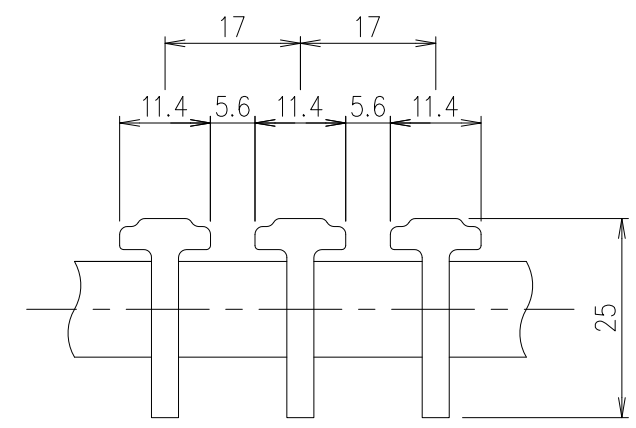
メインバー詳細図 S=1/1
