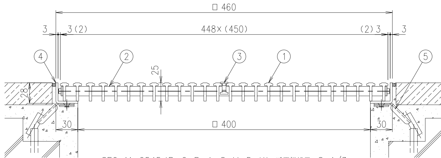
SFG-M-2545 (B・G・P・A・S・M・D・K) 断面詳細図 S=1/3
