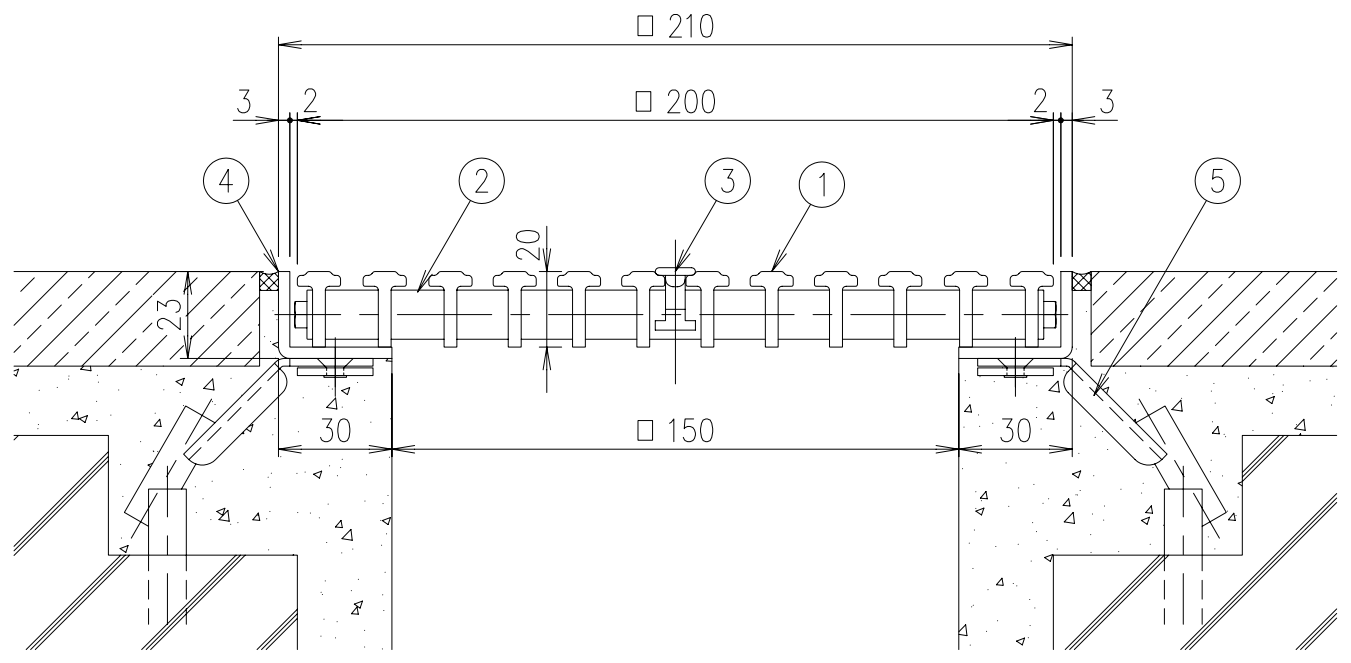
SFG-MF-2020 (B・G・P・A・S・M・D・K) 断面詳細図 S=1/2
