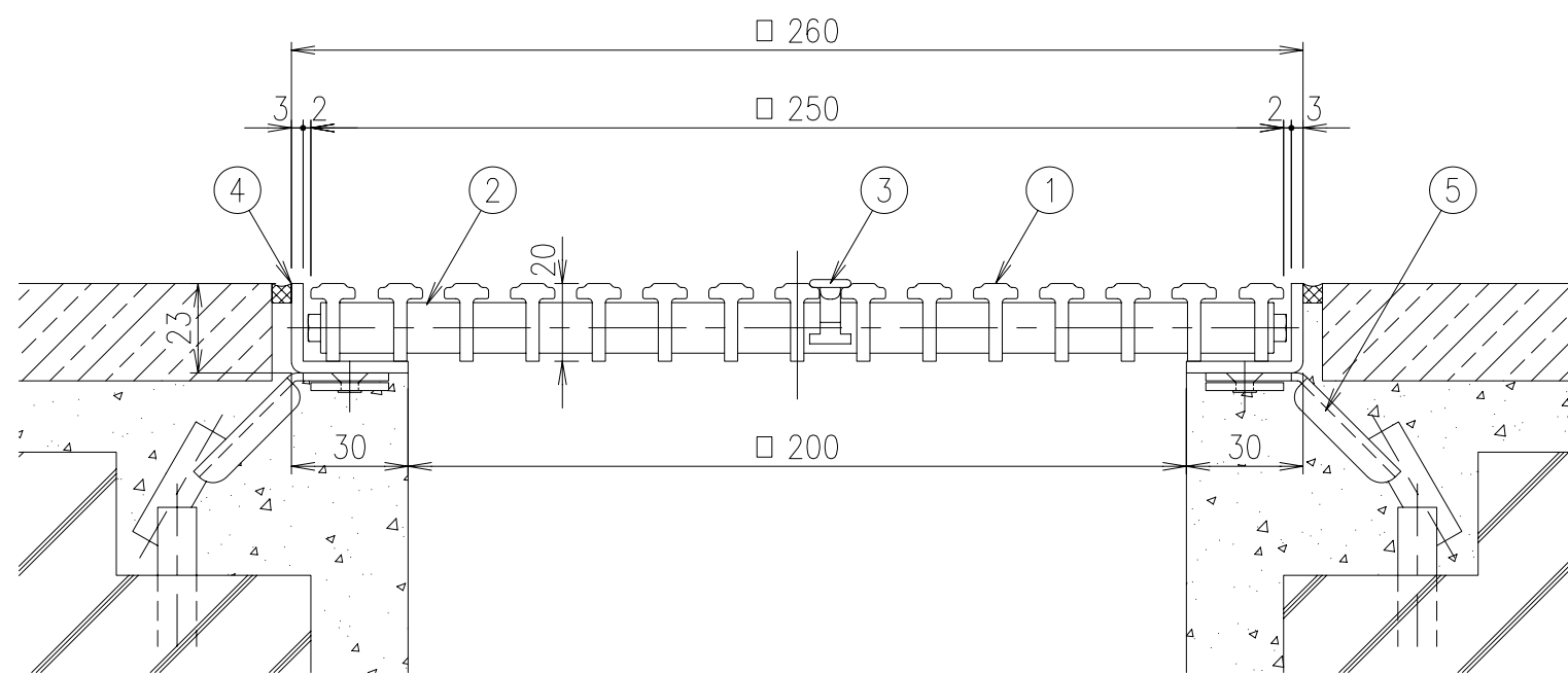
SFG-MF-2025 (B・G・P・A・S・M・D・K) 断面詳細図 S=1/2
