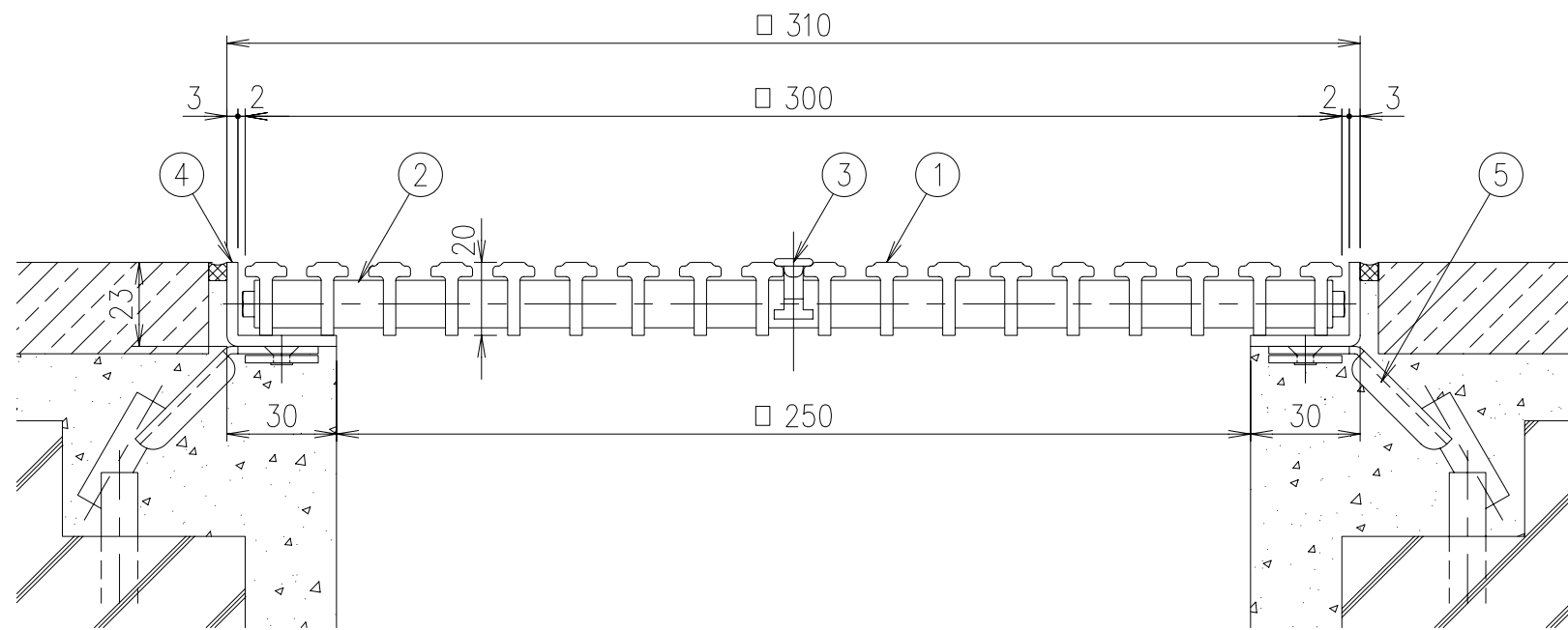
SFG-MF-2030 (B・G・P・A・S・M・D・K) 断面詳細図 S=1/2
