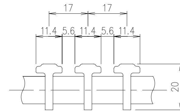
メインバー詳細図 S=1/1
