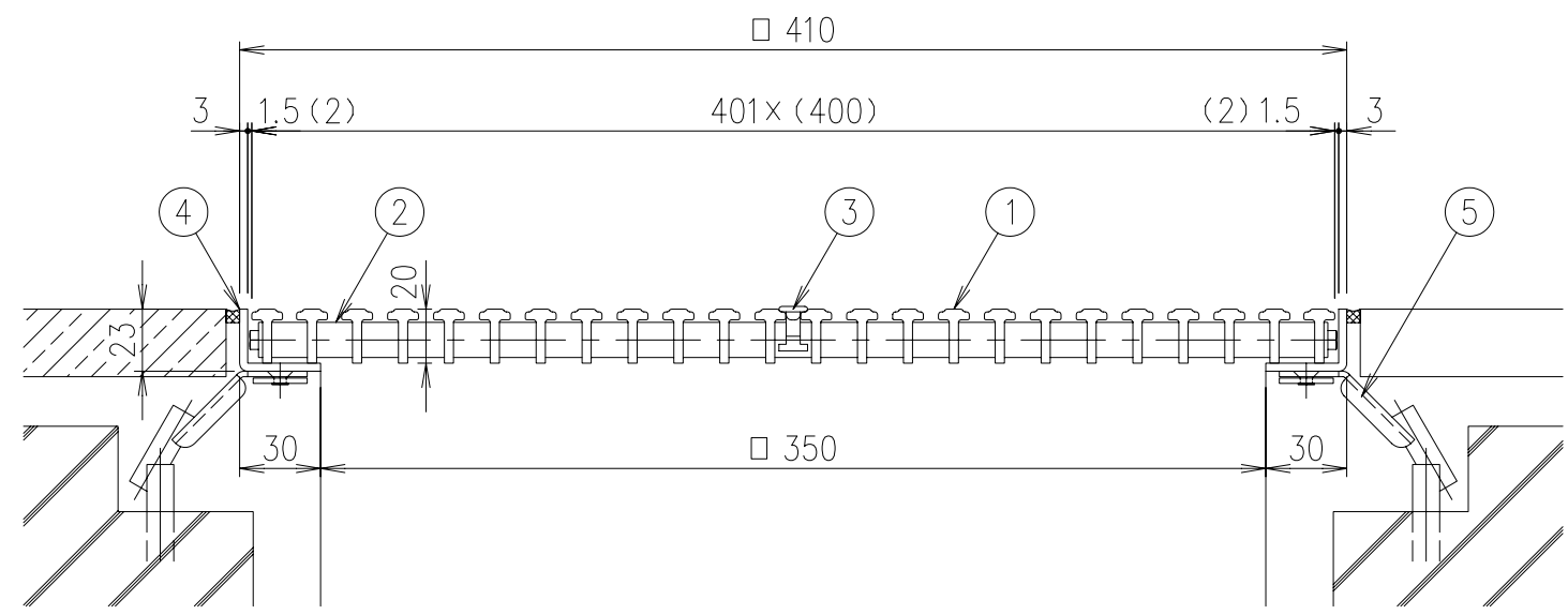
SFG-MF-2040 (B・G・P・A・S・M・D・K) 断面詳細図 S=1/3
