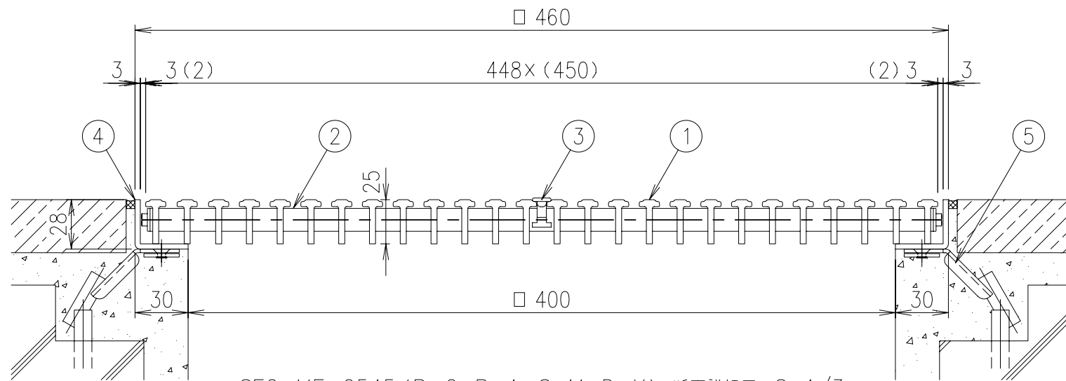
SFG-MF-2545 (B・G・P・A・S・M・D・K) 断面詳細図 S=1/3
