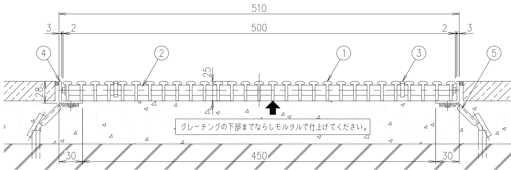
SFG-S-2595 (B・G・P・A・S・M・D・K・C) 断面詳細図 S=1/3
