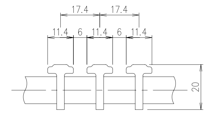
メインバー詳細図 S=1/1
