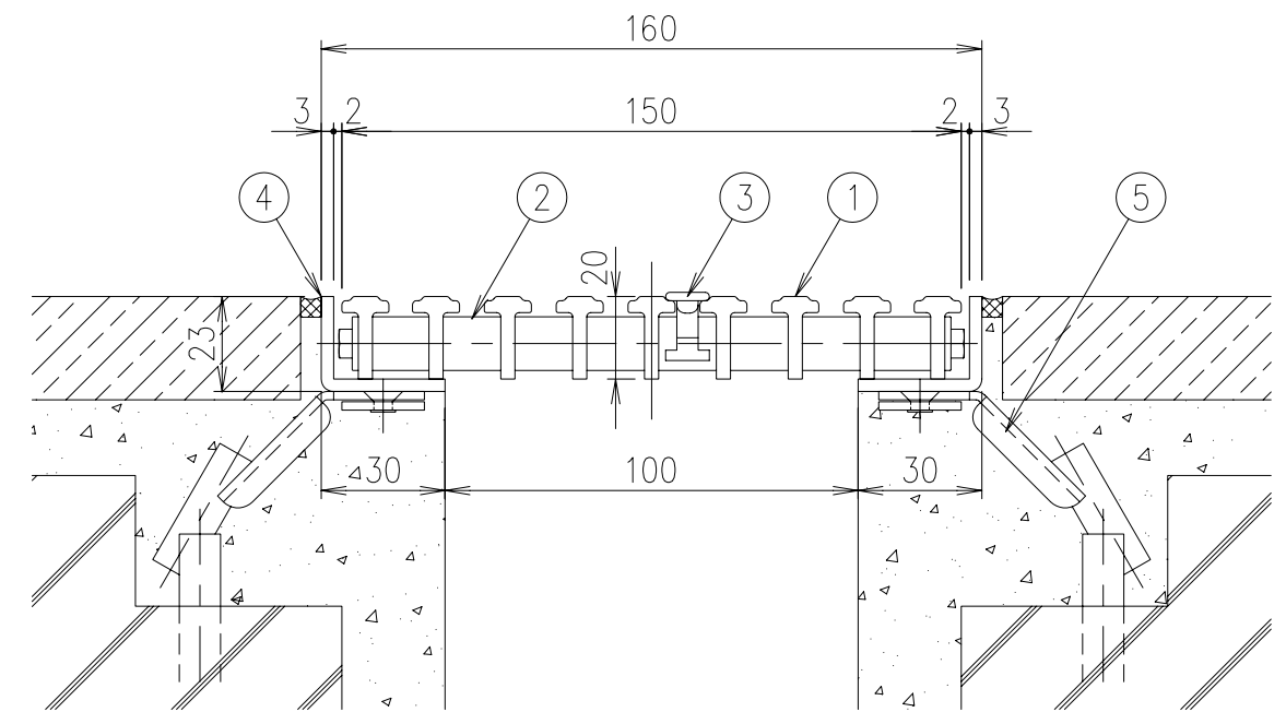
SFG-T-2015 (B・G・P・A・S・M・D・K) 断面詳細図 S=1/2 ◆ ベージュ (B)・ライトグレー (G)・ピンク (P)・ブルー (A)・ホワイト (S) ナチュラルウッド (M)・ダークグレー (D)・ブラック (K) の8色からお選び下さい。
