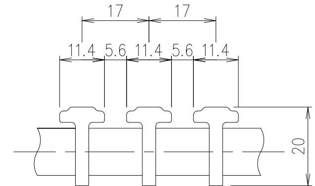
メインバー詳細図 S=1/1
