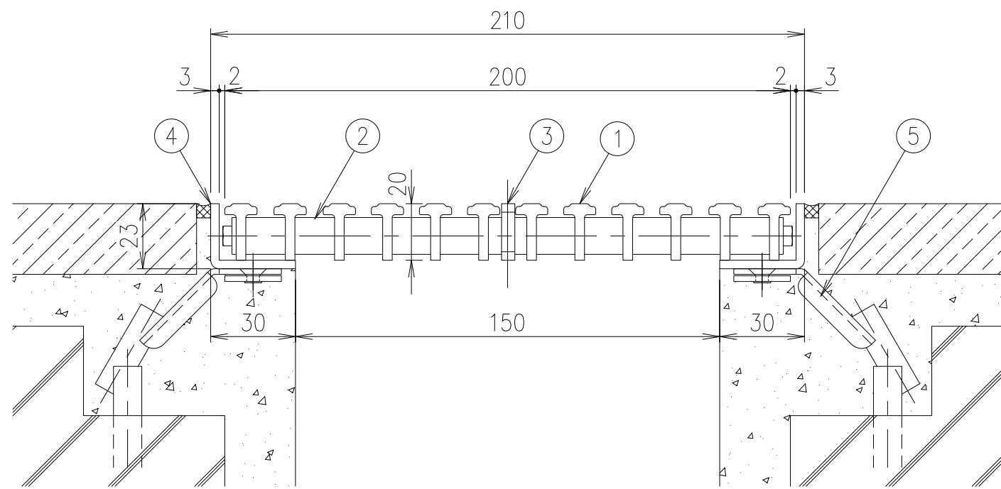
SFG-T-2020 (B・G・P・A・S・M・D・K・C) 断面詳細図 S=1/2 ◆ ページュ (B) ・ライトグレー (G) ・ピンク (P) ・ブルー (A) ・ホワイト (S) ナチュラルウッド (M) ・ダークグレー (D) ・ブラック (K) ・ブラウン (C) の9色からお選び下さい。
