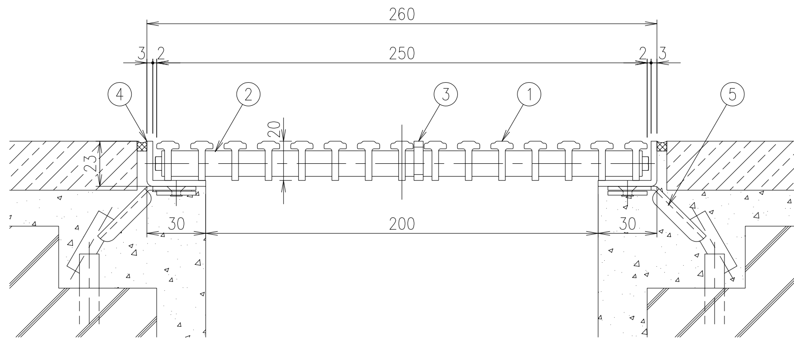
SFG-T-2025 (B・G・P・A・S・M・D・K・C) 断面詳細図 S=1/2 ◆ ベージュ (B)・ライトグレー (G)・ピンク (P)・ブルー (A)・ホワイト (S) ナチュラルウッド (M)・ダークグレー (D)・ブラック (K)・ブラウン (C) の9色からお選び下さい。
