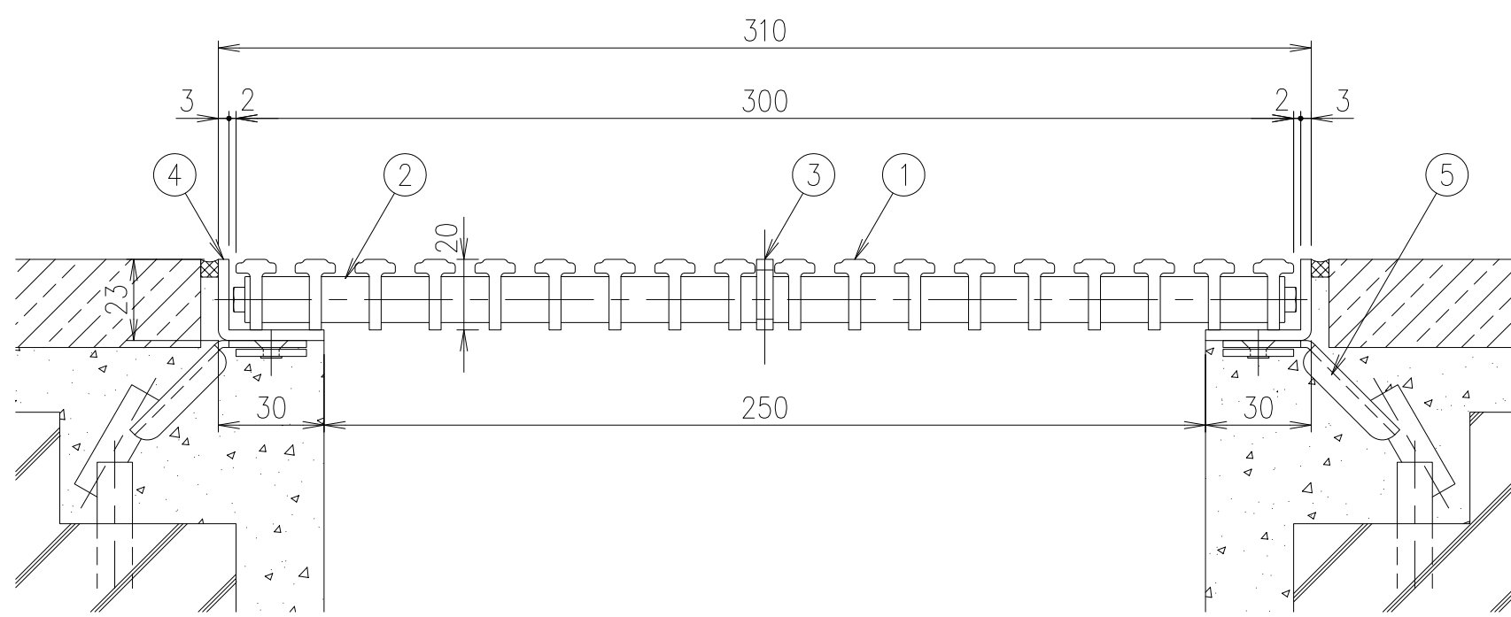
SFG-T-2030 (B・G・P・A・S・M・D・K・C) 断面詳細図 S=1/2 ◆ ベージュ (B)・ライトグレー (G)・ピンク (P)・ブルー (A)・ホワイト (S) ナチュラルウッド (M)・ダークグレー (D)・ブラック (K)・ブラウン (C) の9色からお選び下さい。
