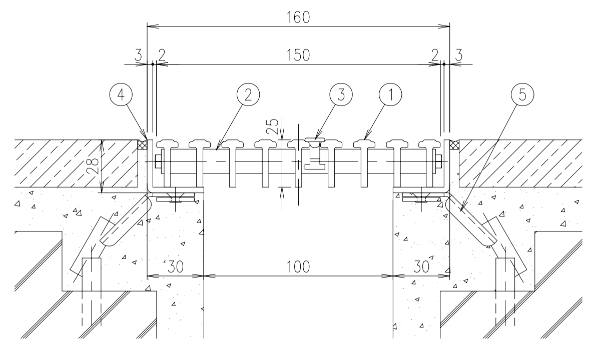
SFG-T-2515 (B・G・P・A・S・M・D・K) 断面詳細図 S=1/2 ◆ ベージュ (B)・ライトグレー (G)・ピンク (P)・ブルー (A)・ホワイト (S) ナチュラルウッド (M)・ダークグレー (D)・ブラック (K) の8色からお選び下さい。
