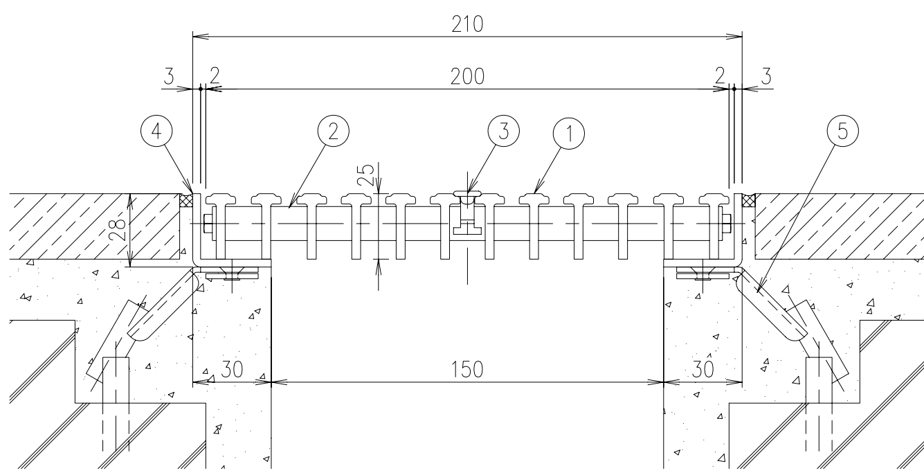
SFG-T-2520 (B・G・P・A・S・M・D・K) 断面詳細図 S=1/2 ◆ ベージュ (B)・ライトグレー (G)・ピンク (P)・ブルー (A)・ホワイト (S) ナチュラルウッド (M)・ダークグレー (D)・ブラック (K) の8色からお選び下さい。
