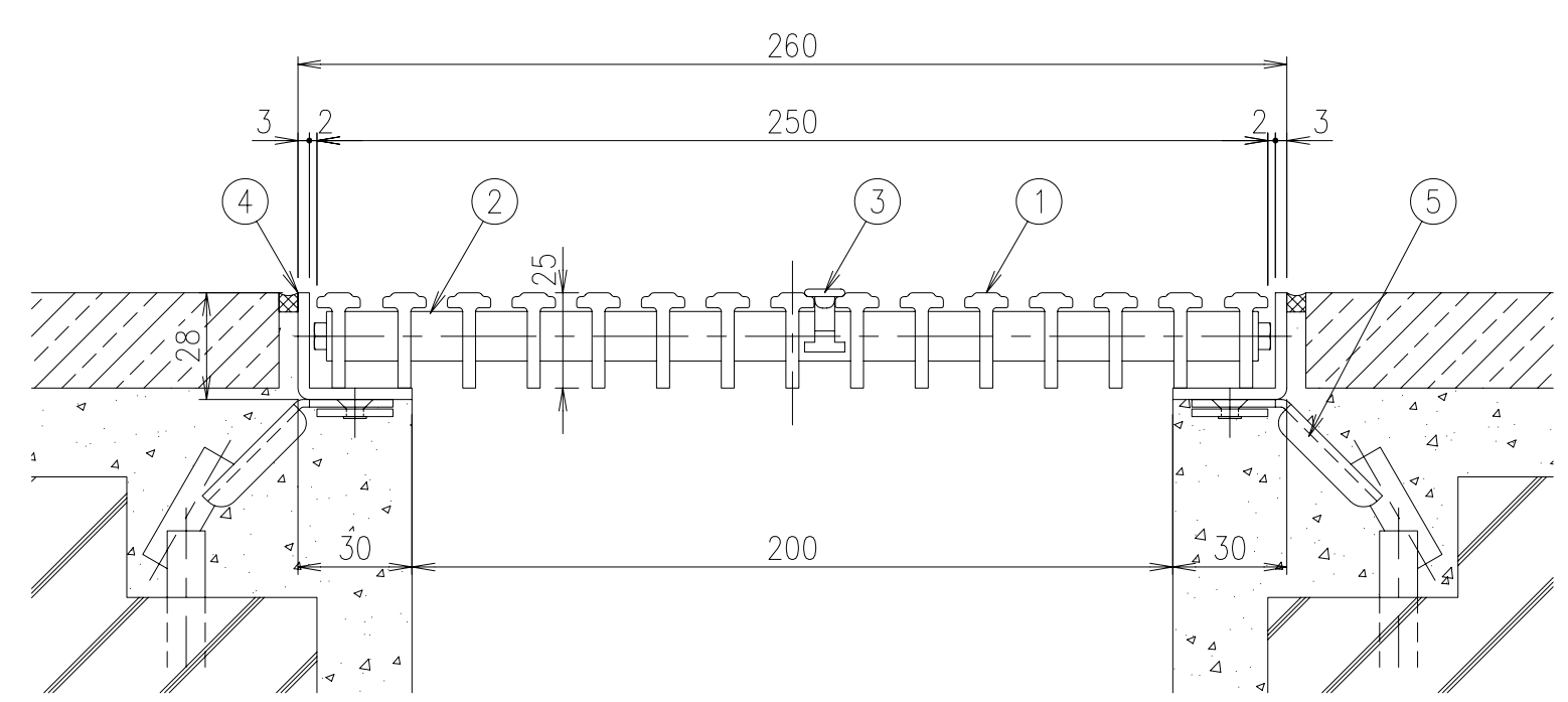
SFG-T-2525 (B・G・P・A・S・M・D・K) 断面詳細図 S=1/2 ◆ ベージュ (B)・ライトグレー (G)・ピンク (P)・ブルー (A)・ホワイト (S) ナチュラルウッド (M)・ダークグレー (D)・ブラック (K) の8色からお選び下さい。
