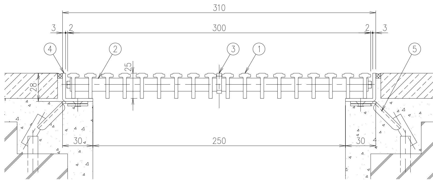
SFG-T-2530 (B・G・P・A・S・M・D・K・C) 断面詳細図 S=1/2 ◆ ベージュ (B)・ライトグレー (G)・ピンク (P)・ブルー (A)・ホワイト (S) ナチュラルウッド (M)・ダークグレー (D)・ブラック (K)・ブラウン (C) の9色からお選び下さい。
