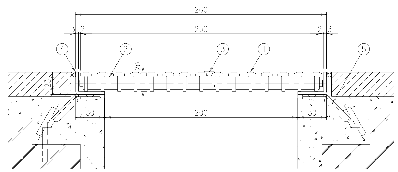
SFG-TF-2025 (B・G・P・A・S・M・D・K) 断面詳細図 S=1/2 ◆ ベージュ (B)・ライトグレー (G)・ピンク (P)・ブルー (A)・ホワイト (S) ナチュラルウッド (M)・ダークグレー (D)・ブラック (K) の8色からお選び下さい。
