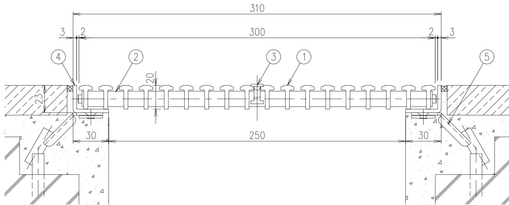
SFG-TF-2030 (B・G・P・A・S・M・D・K) 断面詳細図 S=1/2 ◆ ベージュ (B)・ライトグレー (G)・ピンク (P)・ブルー (A)・ホワイト (S) ナチュラルウッド (M)・ダークグレー (D)・ブラック (K) の8色からお選び下さい。
