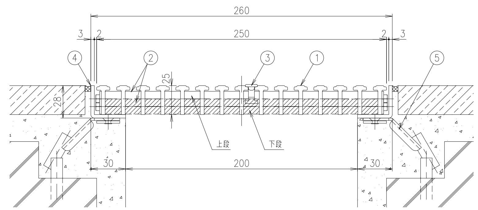
SFG-TF-2525 (B・G・P・A・S・M・D・K) 断面詳細図 S=1/2 ◆ ベージュ (B) ・ライトグレー (G) ・ピンク (P) ・ブルー (A) ・ホワイト (S) ・ナチュラルウッド (M) ・ダークグレー (D) ・ブラック (K) の8色からお選び下さい。
