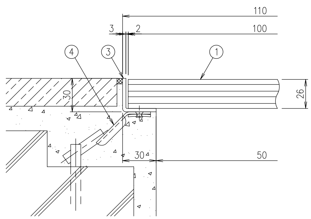
SFG-10 断面詳細図 S=1/2
