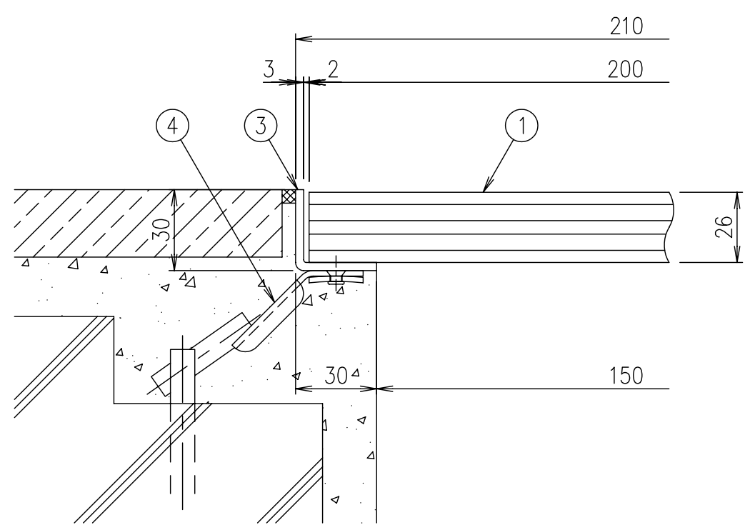
SFG-20 断面詳細図 S=1/2
