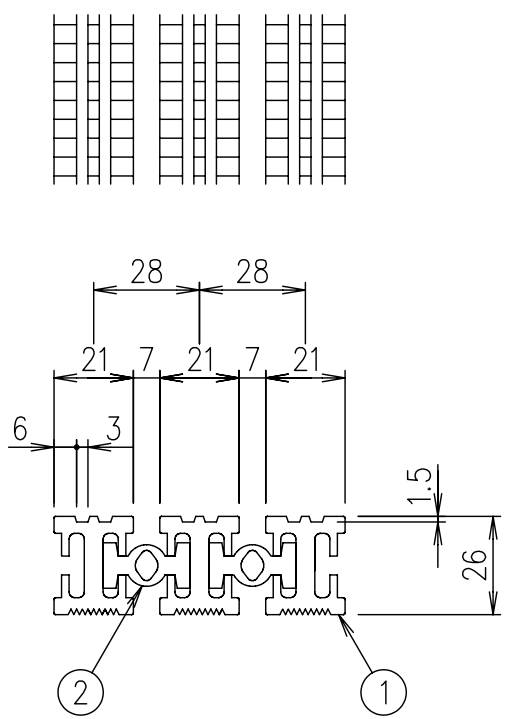
メインバー詳細図 S=1/2
