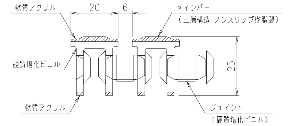
A部拡大図 S=1/1
