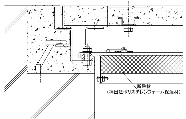
トレンチピット蓋仕様例 (T-20 みぞ幅 600mm用)
