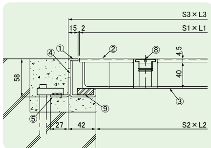
●断面図 BH-CS
