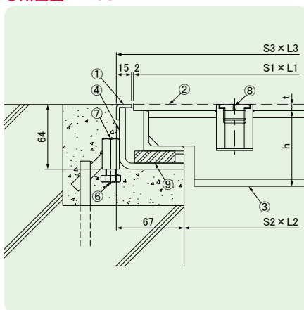
●断面図 BH-CS-14
