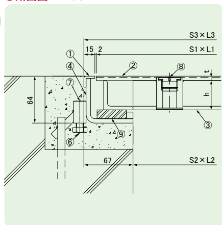
●断面図 BH-CS-2
