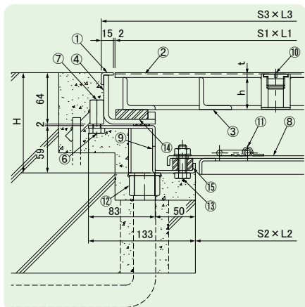
●断面図 BH-CSW-2
