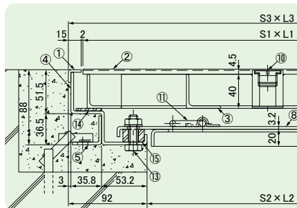
●断面図 BH-CSW
