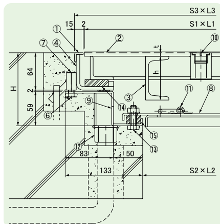
●断面図 BH-CSW-14
