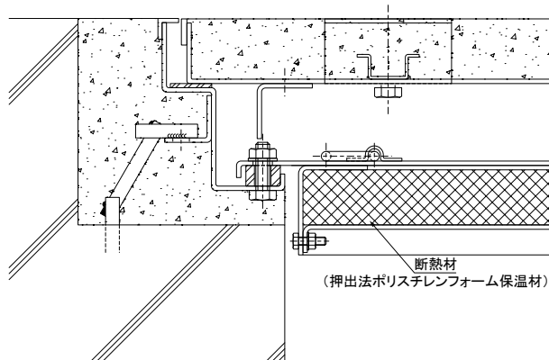
トレンチピット蓋仕様例 (T-20 みぞ幅 600mm用)
