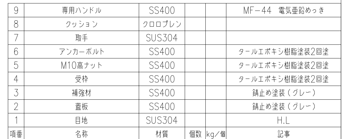
記号 内容 日付 編集 担当 製図 照査 承認 1 10 名称 DKC 坂本 菅原 気田 尺度 縞鋼板マシンハッチ BH-CS-14 800×800 (T-14) 年 月 日 三角法 図番 B-E3-05799 第一機材株式会社 親番 図歴
