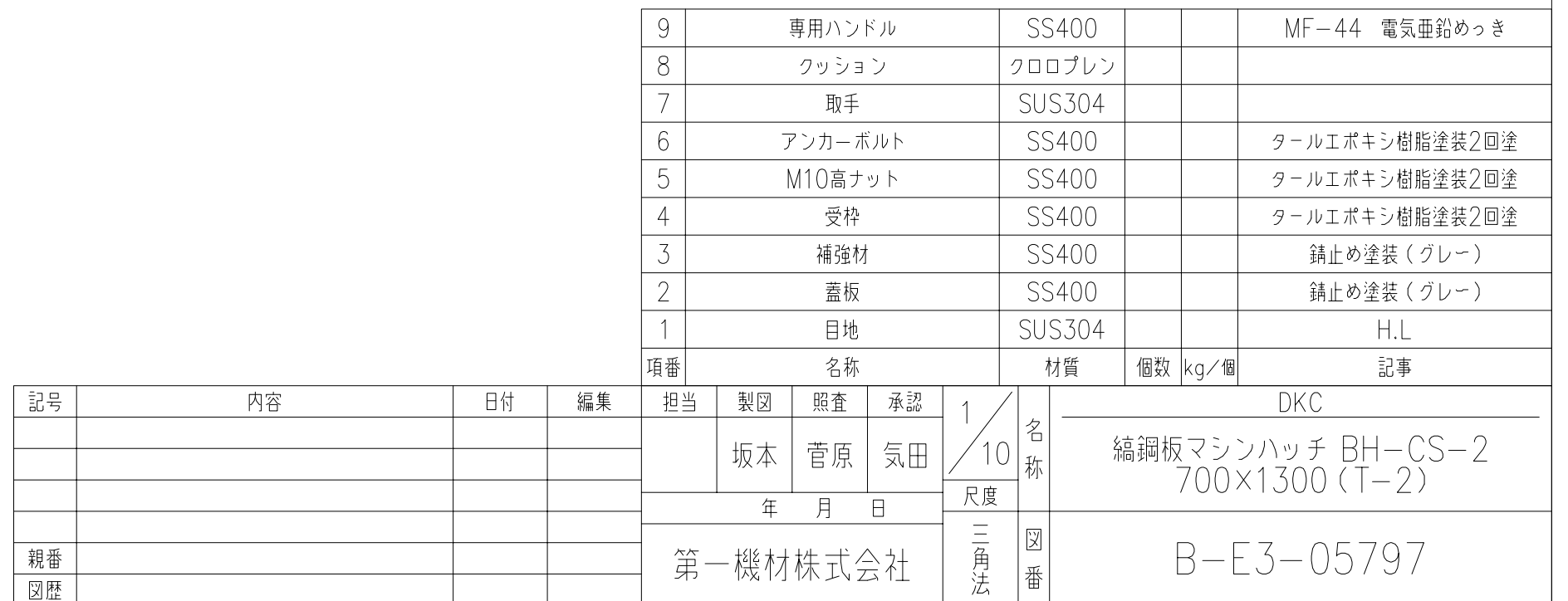
計算重量 蓋：約28kg/枚 受枠：約30kg
