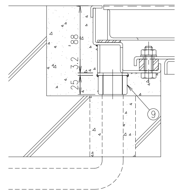
ソケット部詳細図 S=1/3
