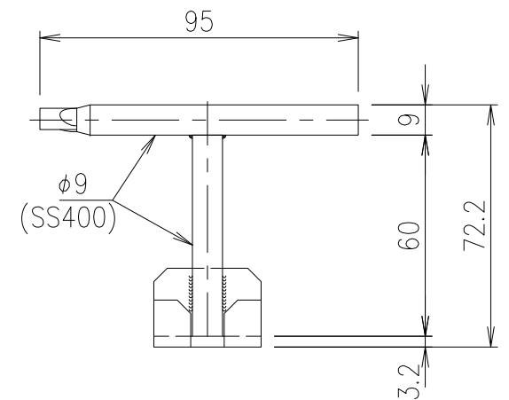
⑦ 専用ハンドル S=1/2
