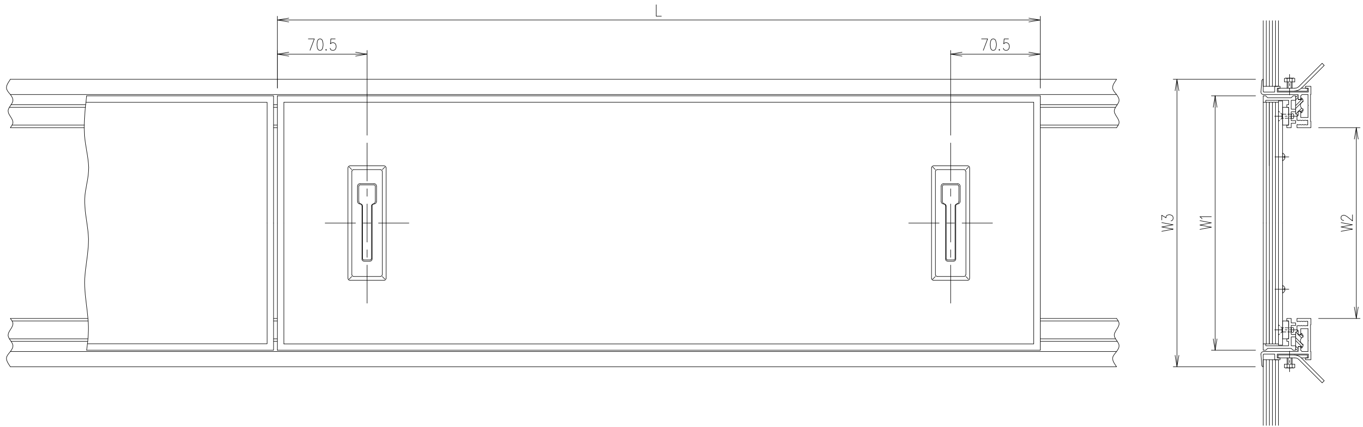
寸 法 表 単位：mm
