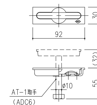
取手(AT-1) 詳細図 S=1/3 ※取手はオプション部品です
