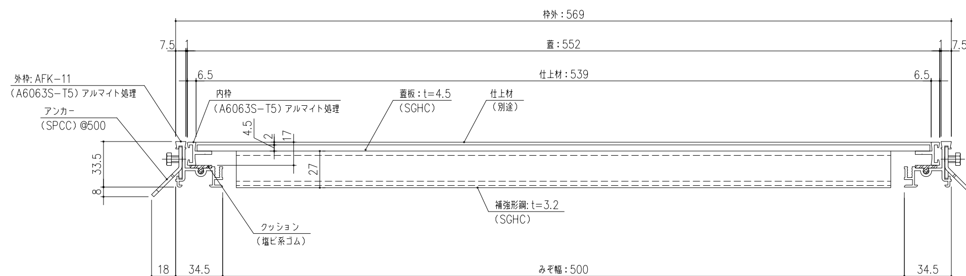
AP2-T4-55 断面詳細図 S=1/2 貼物用 配線ピット蓋 ※荷重条件：歩行用(3.5kN/m 2 )
