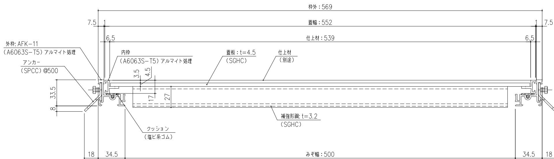
AP3-T4-55 断面詳細図 S=1/2 貼物用 配線ピット蓋 ※荷重条件：歩行用 (3.5KN/m 2 )
