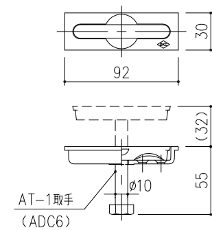
取手(AT-1) 詳細図 S=1/3
