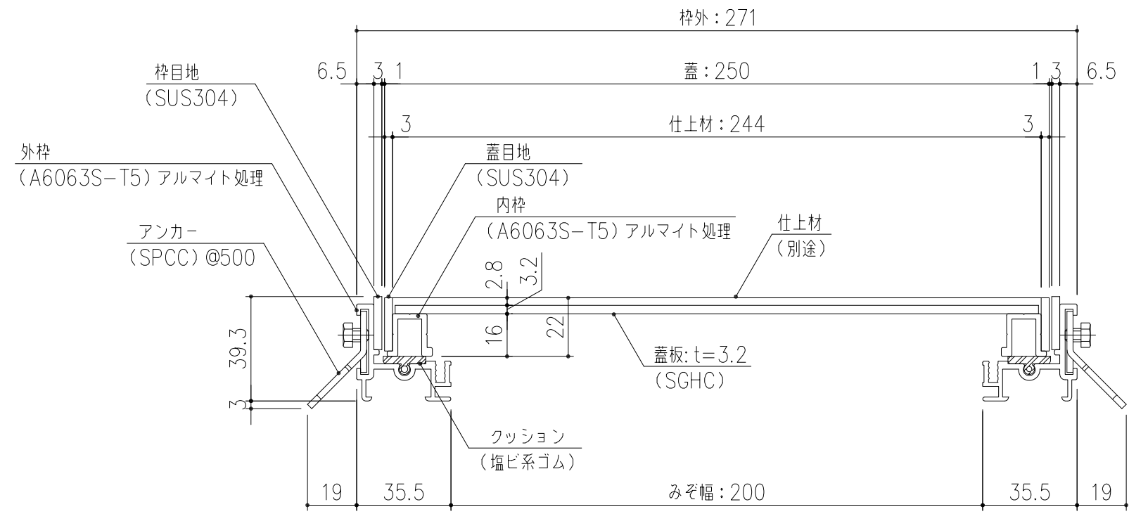
SP3-T3-25 断面詳細図 S=1/2 貼物用配線ピット蓋 ※荷重条件：歩行用 (3.5KN/m 2 )
