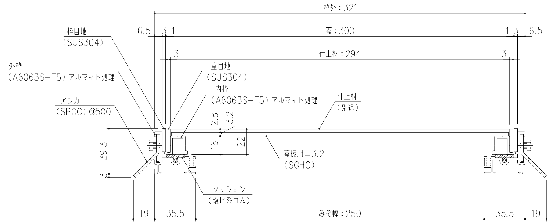
SP3-T3-30 断面詳細図 S=1/2 貼物用配線ピット蓋 ※荷重条件：歩行用 (3.5KN/m 2 )
