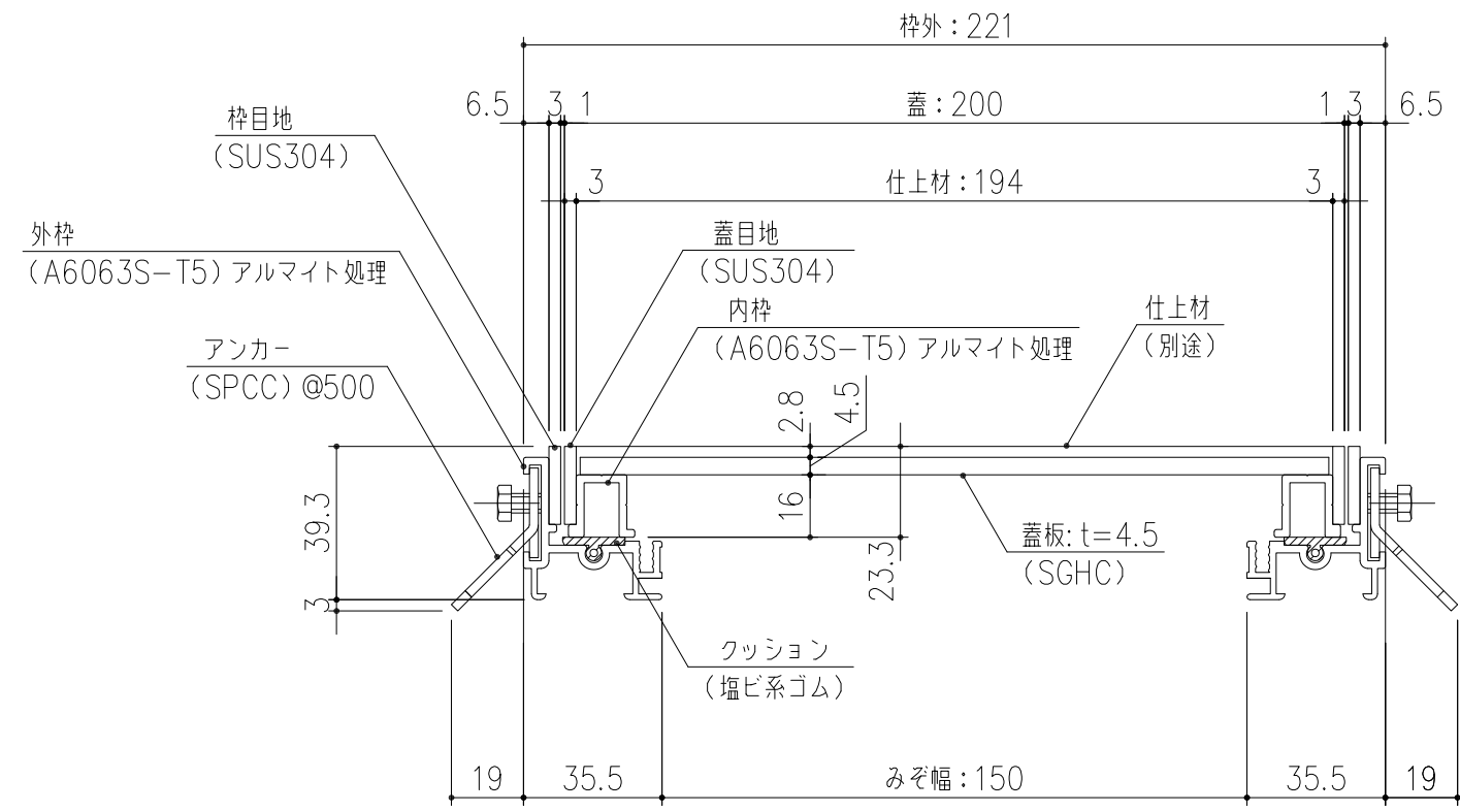
SP3-T4-20 断面詳細図 S=1/2 貼物用配線ピット蓋 ※荷重条件: 歩行用 (3.5KN/m 2 )
