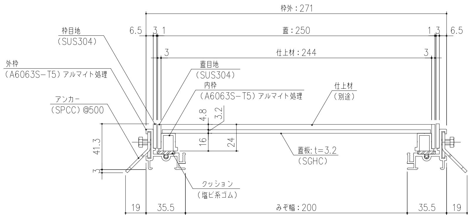
SP5-T3-25 断面詳細図 S=1/2 貼物用配線ピット蓋 ※荷重条件: 歩行用 (3.5KN/m 2 )
