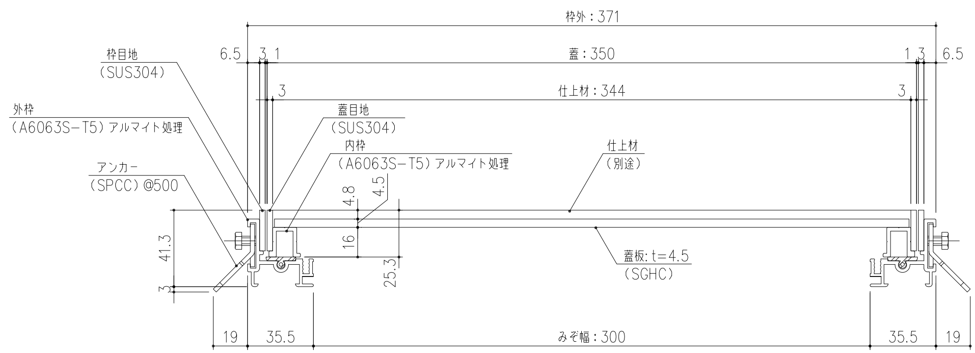
SP5-T4-35 断面詳細図 S=1/2 貼物用配線ピット蓋 ※荷重条件：歩行用 (3.5KN/m 2 )
