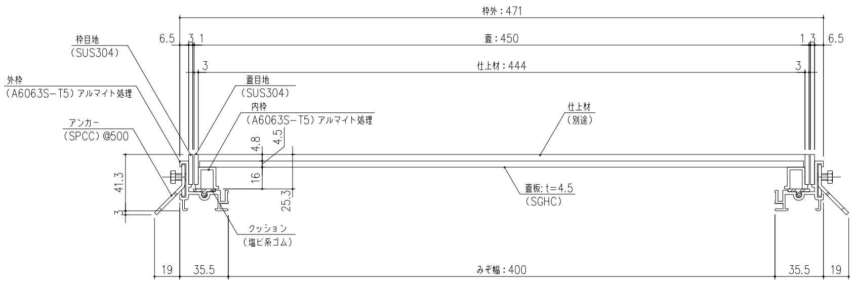
SP5-T4-45 断面詳細図 S=1/2 貼物用配線ビット蓋 ※荷重条件：歩行用 (3.5KN/m 2 )
