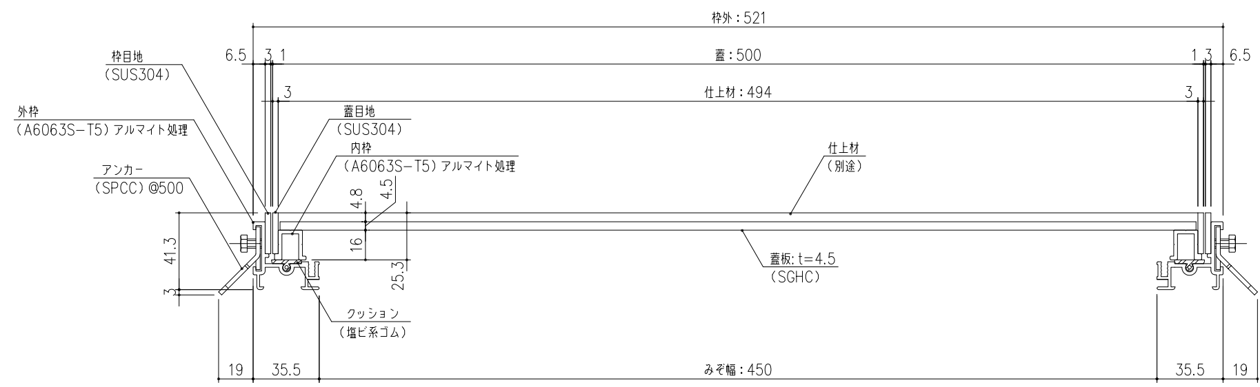
SP5-T4-50 断面詳細図 S=1/2 貼物用配線ピット蓋 ※荷重条件：歩行用 (3.5KN/m 2 )
