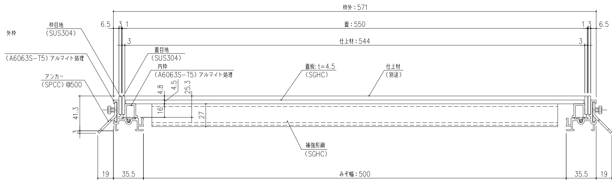
SP5-T4-55 断面詳細図 S=1/2 貼物用配線ビット蓋 ※荷重条件: 歩行用 (3.5KN/m 2 )
