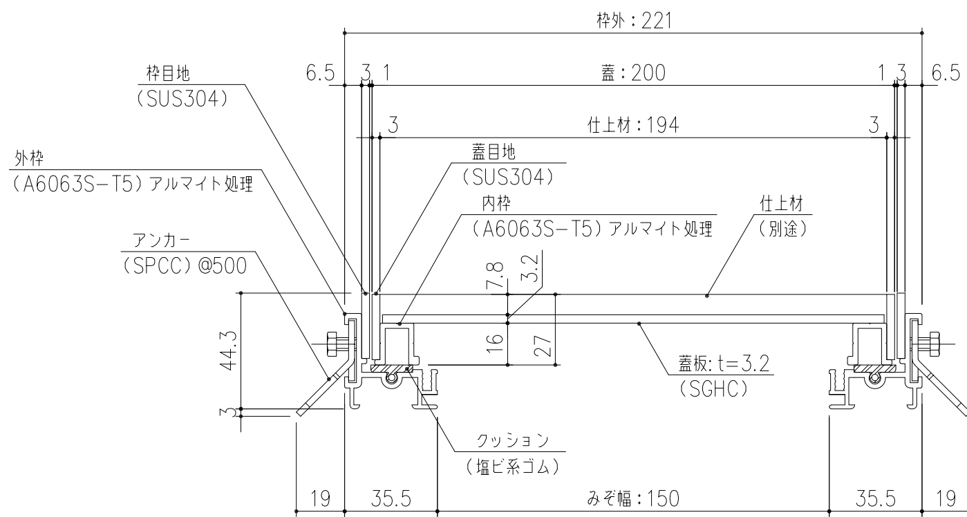
SP7-T3-20 断面詳細図 S=1/2 貼物用配線ピット蓋 ※荷重条件: 歩行用 (3.5KN/m 2 )
