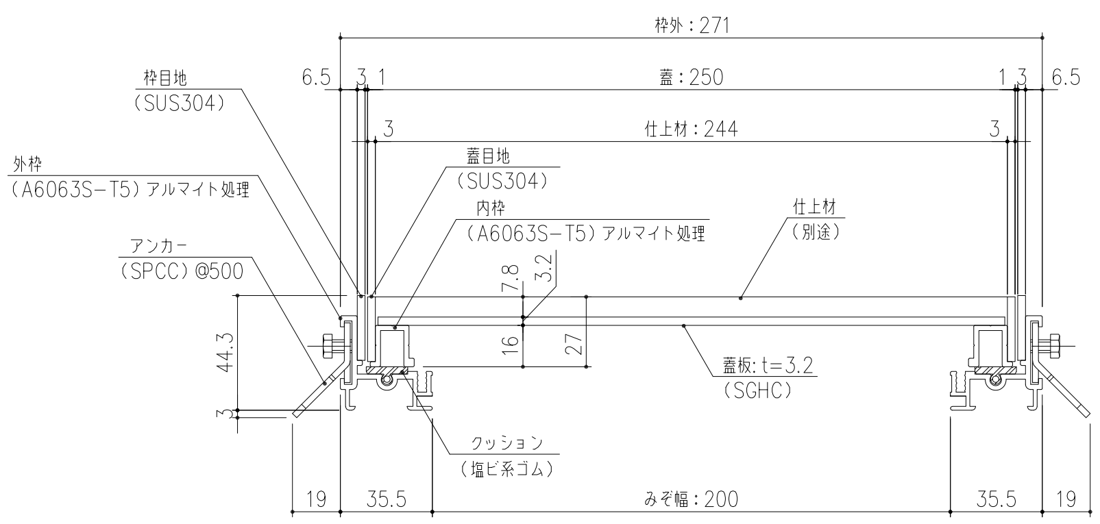
SP7-T3-25 断面詳細図 S=1/2 貼物用配線ピット蓋 ※荷重条件: 歩行用 (3.5KN/m 2 )
